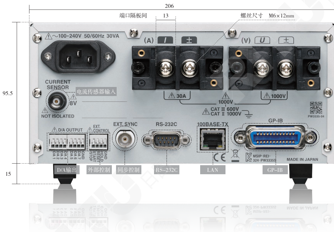
PW3335-04背面图
