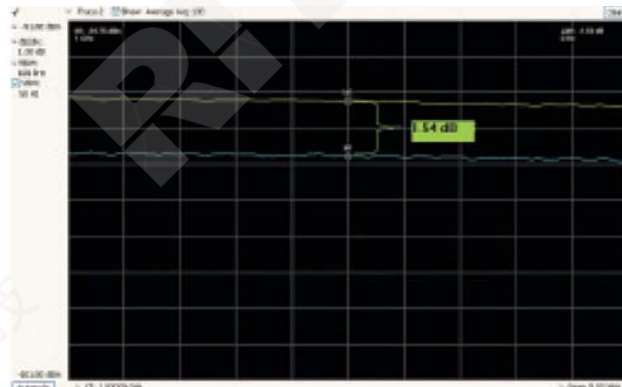
图 4. 使用 100 kHz 滤波器测量的随机噪声。-3dB, 100 kHz 响应用黄色表示，-6dB, 100 kHz 响应用蓝色表示。功率差是 1.54 dB，与理论值非常接近。
