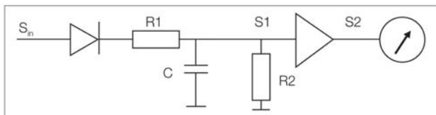
图5. 模拟实现方案中的准峰值检测器。准峰值检测器的响应快(充电时间)、衰减慢(放电时间)特点源于这条电路中实现的 R-C 常数。得到的波形驱动着临界阻尼表。
