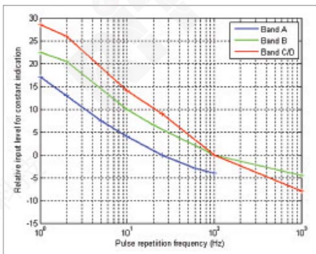
图7. 准峰值检测器的脉冲响应曲线。
