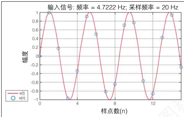
图 2-12. 输入信号。
