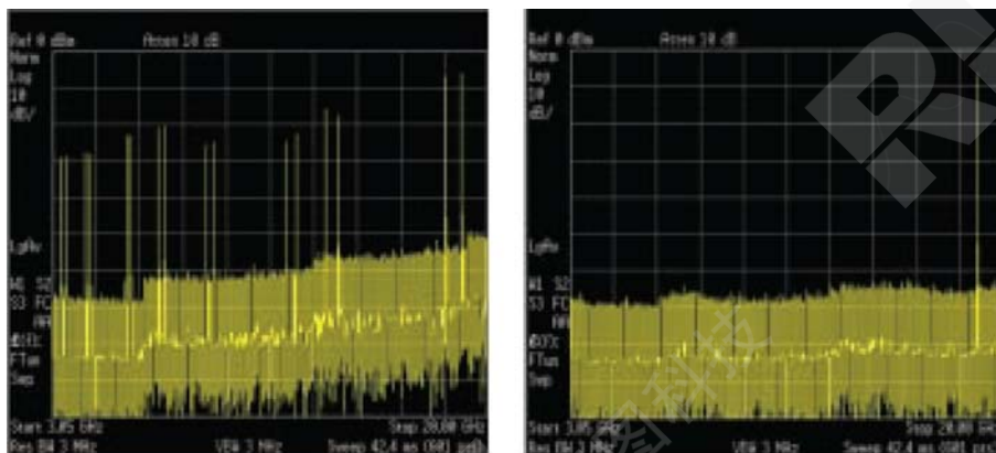
图 2-2. (左) 这是在去掉 YIG 预选滤波器时传统频谱分析仪微波频率范围内可以表示的典型的单个信号。(右) 恢复预选滤波器，然后可以显示单个信号。
