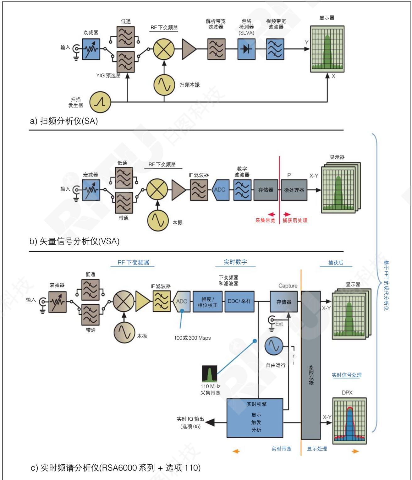
图 1-2 a, b, c: 扫频分析仪(a)、矢量信号分析仪(b)和实时频谱分析仪(c)简化的方框图。
