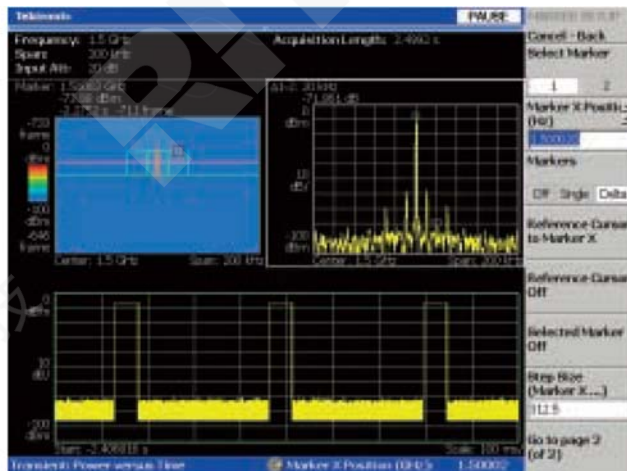
图 3-24. 多域视图，显示频谱图、功率随频率变化及功率随时间变化。
