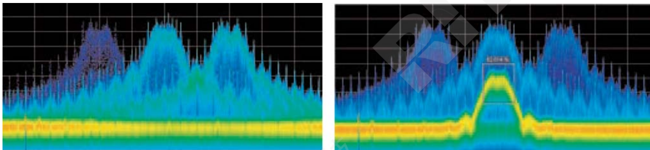
图 2-27. 密度触发功能实例。左：自由运行的 DPX 频谱画面，显示脉冲随频率变化。中间的短脉冲偶尔会在瞬间出现，但仅仅使用 Run/Stop 按钮很难捕获到。右：已触发的 DPX 画面，显示未触发的画面中没有显现的低幅度脉冲。分析仪被设置在用户画的框中的平均密度达到 50% 或以上时触发。
