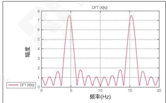
图 2-13. 连续求解 x(n) 的 DFT。
