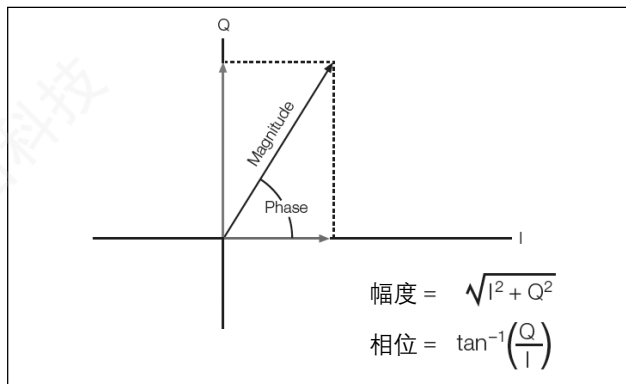
图 2-35. 幅度和相位的矢量表示。
