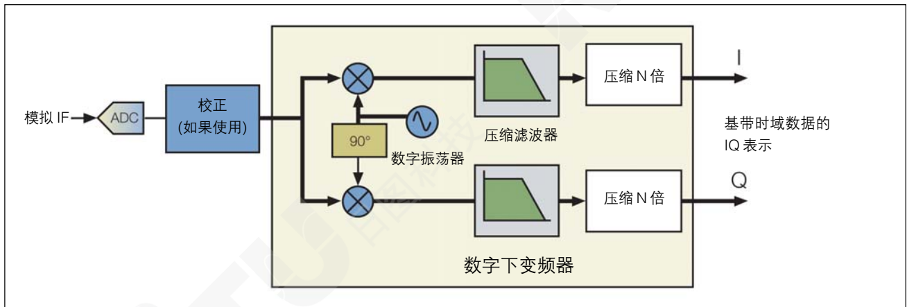
图 2-4: 实时频谱分析仪中的 IF 到 IQ 转换。
