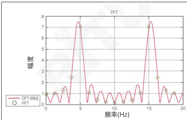
图 2-14. x(n) 的 FFT, FFT 的长度 =N=x(n) 的长度。
