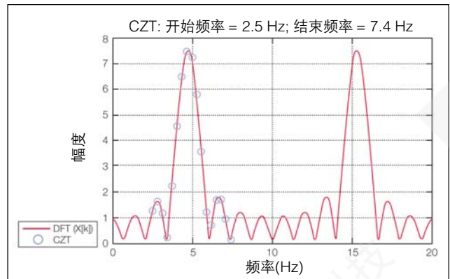
图 2-15. x(n) 的 CZT。
