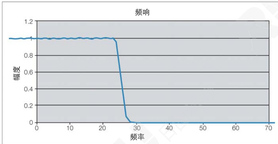
图 2-16. 低通滤波器的频响。
