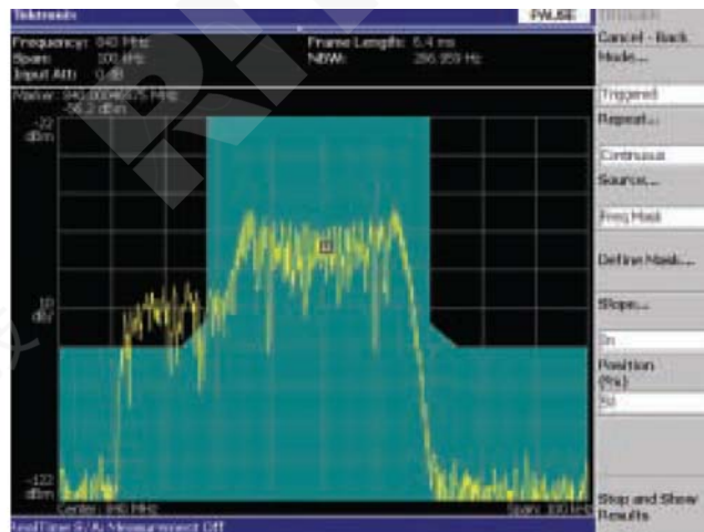
图2-34. 频谱图的一个帧，显示了瞬时信号越过频率模板边界的瞬时事件。
