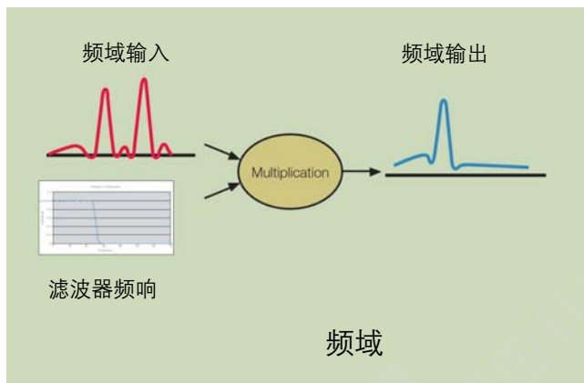
图 2-18. 滤波器乘以频响。
