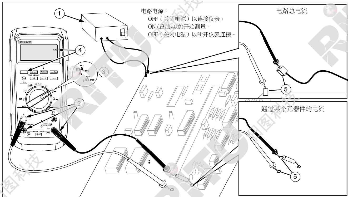
图 3 电流测量
