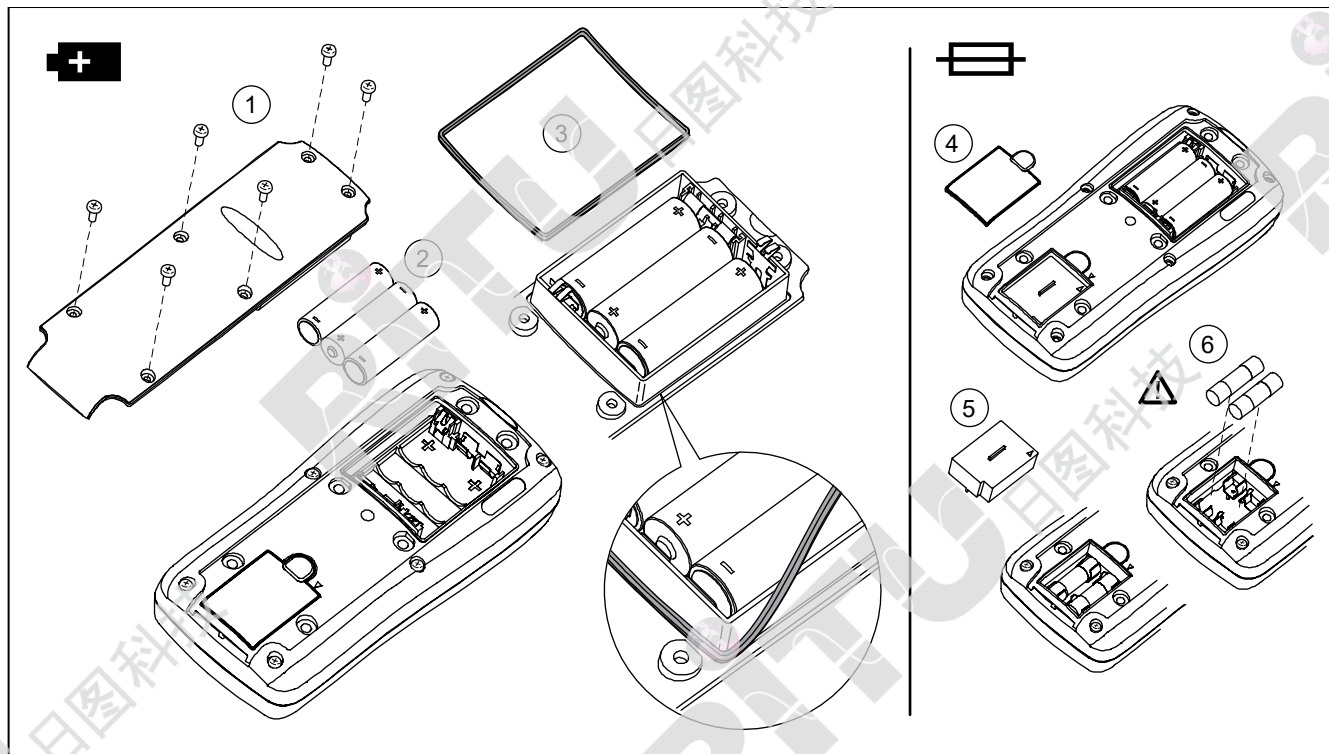
图 11. 电池和保险丝更换
