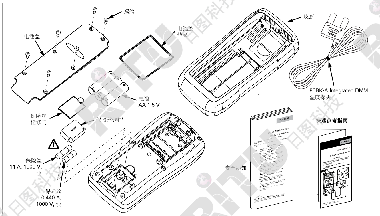
图 12.可换部件
