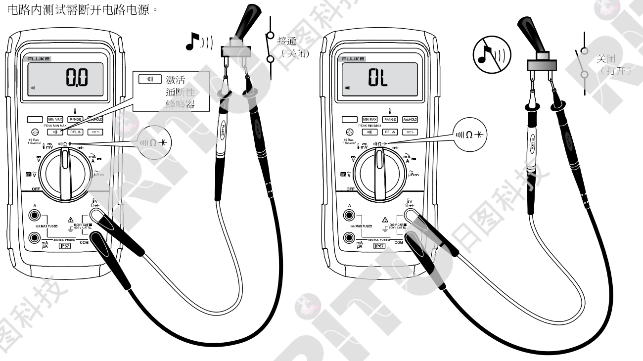
图 4. 通断性测试
