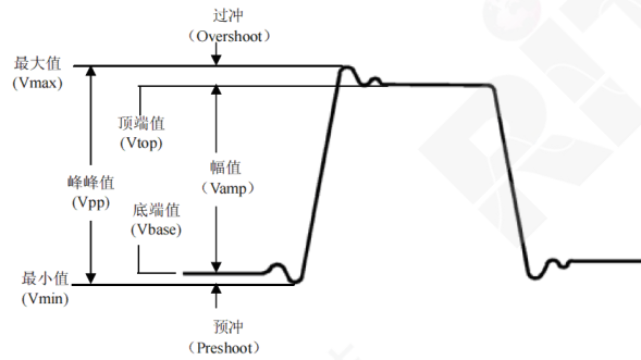
图 7-2 电压参数示意图
