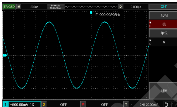
图 2-8 垂直通道反相设置(未反相)
