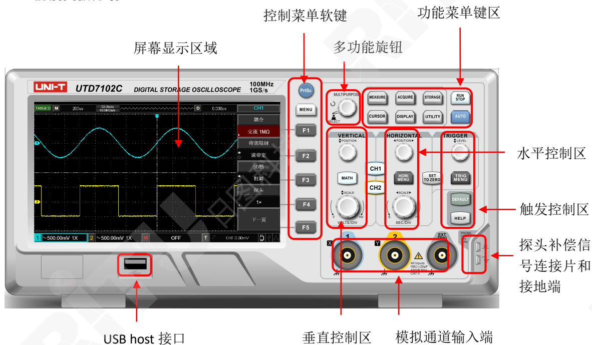
图 1-3 示波器前面板
