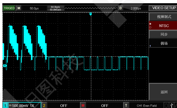
图 4-2 视频场同步
