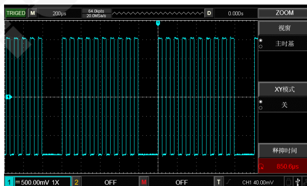
图 4-4 使用触发释抑同步复杂波形
