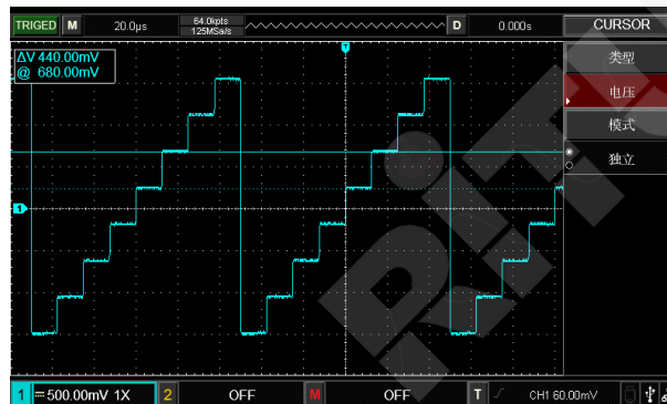
图 12-6 光标测量信号电压差
