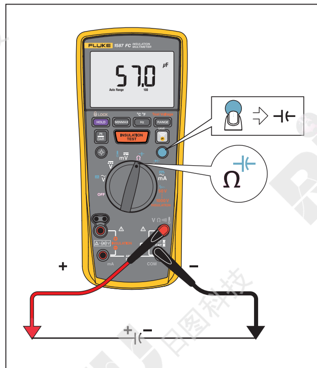
图 5. 测量电容
