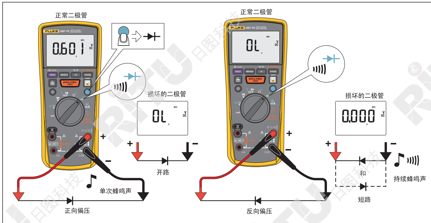
图 7. 测试二极管
