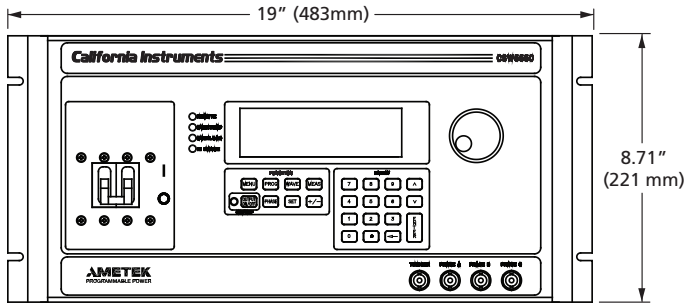
正视图
