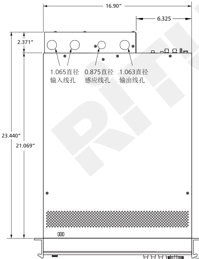
俯视图
