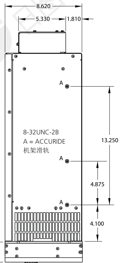
侧视图
