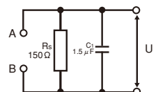
● 测量回路网(网络PCC-2 IEC60598-1)
