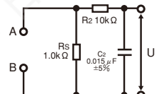
● 测量回路网(网络I IEC60601-1等)
