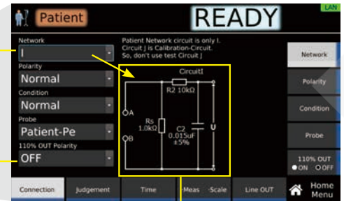
测量网络显示(网络 I IEC60601-1)
