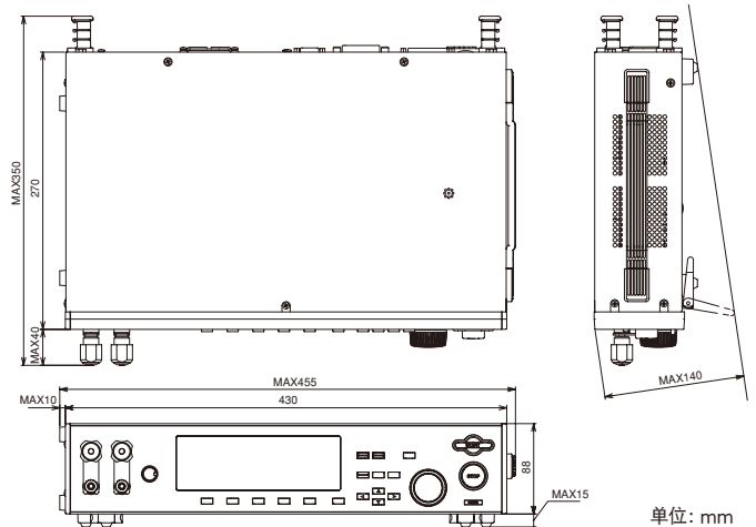
—外形尺寸图—
