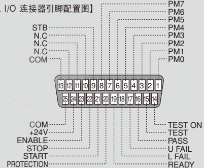
【SIGNAL I/O 连接器引脚配置图】
