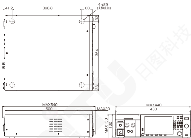
TOS9302 TOS9303
