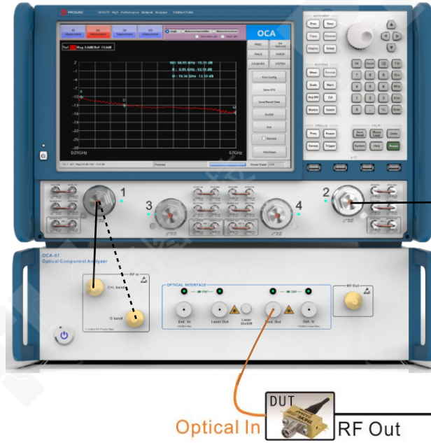
Single-ended 光电器件测量 待测件连接示意图
