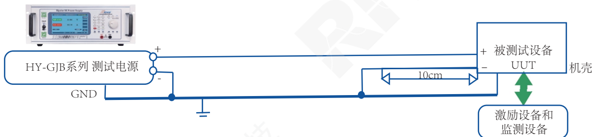
图LDC201-1 供电转换中断试验系统典型配置
