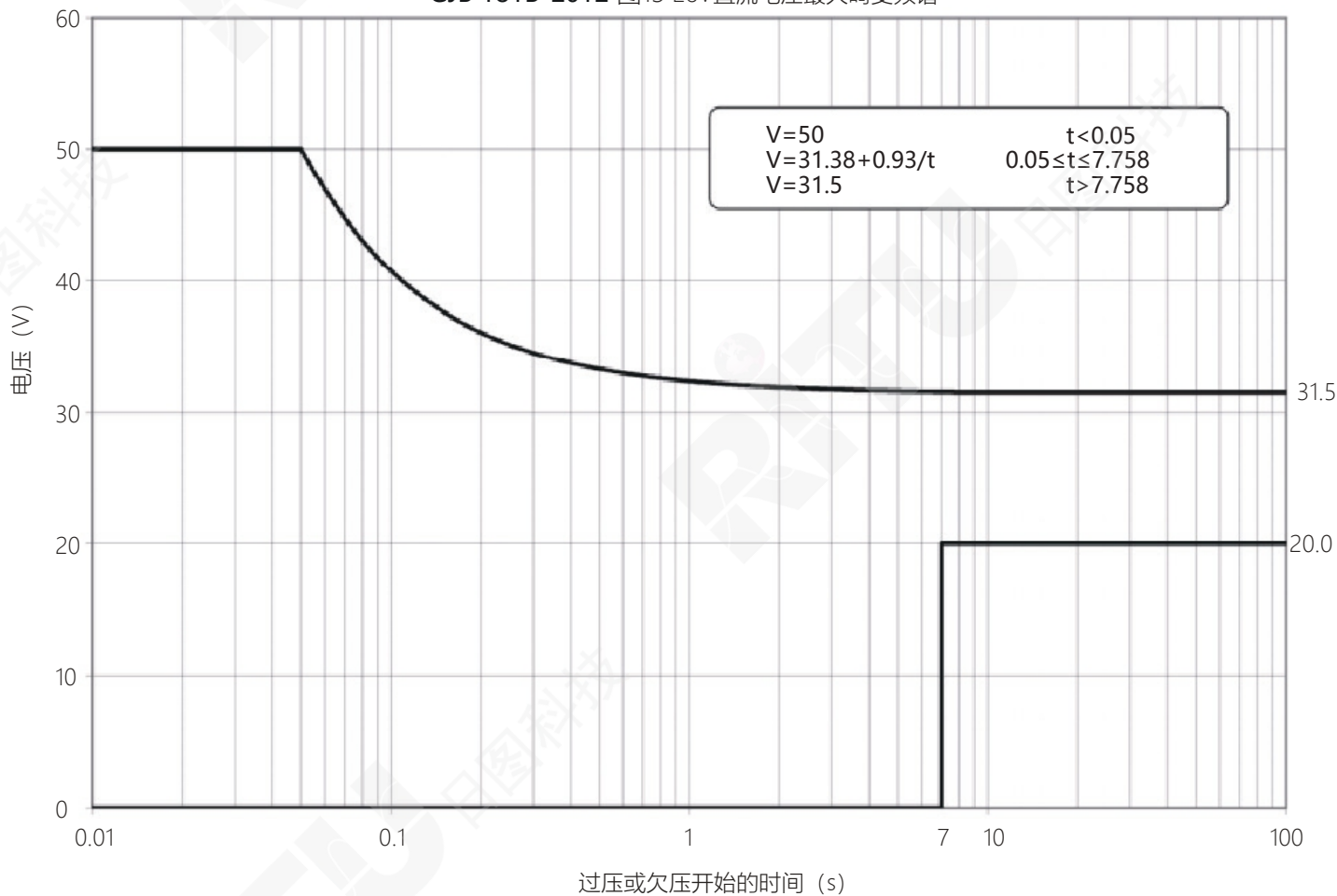
GJB 181B-2012 图14 28V直流非正常工作电压极限
