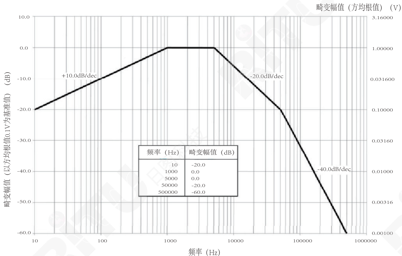
GJB 181B-2012 图13 28V直流电压最大畸变频谱
