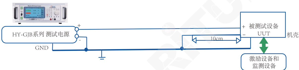
图LDC301-1 非正常稳态电压试验条件
