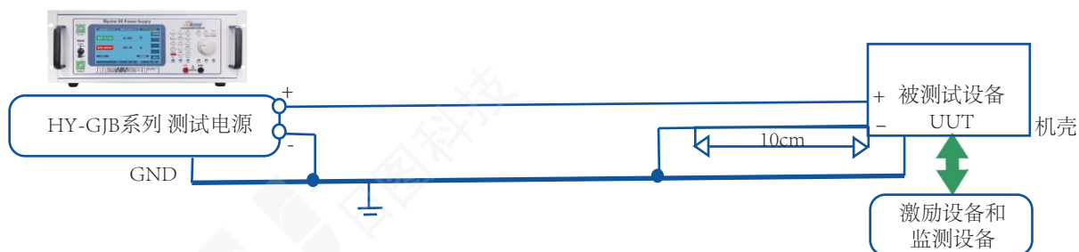
图LDC101-1 负载特性试验系统典型配置
