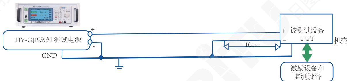
图LDC601-1 断电试验系统典型配置
